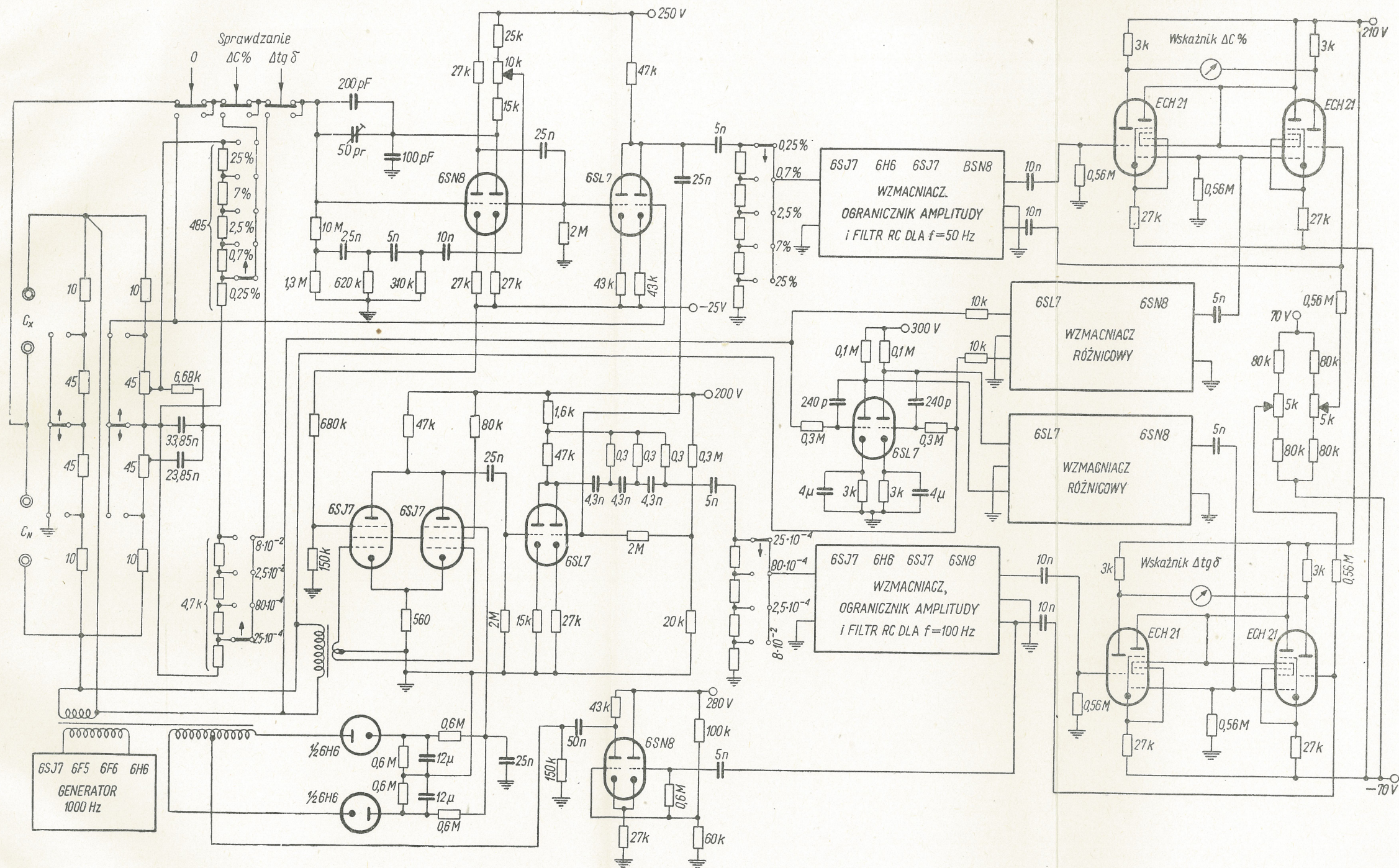
Rys. 13. Uproszczony schemat przyrządu do odchyłowych pomiarów własności elektrycznych kondensatorów
